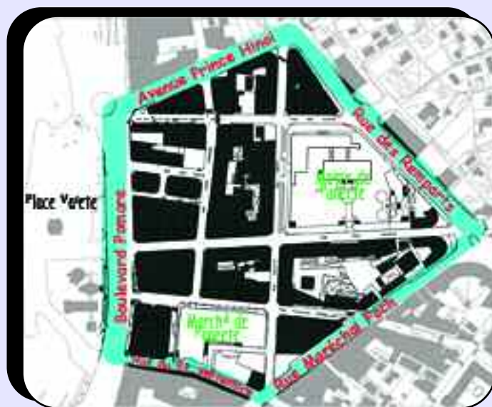
Plan de situation de la zone couverte par la collecte des eaux usées de la station d'épuration communale située à l'Hôtel de ville
